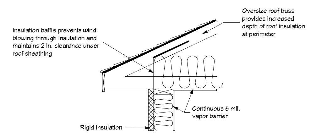
6 OPTIONAL EAVE DETAIL
